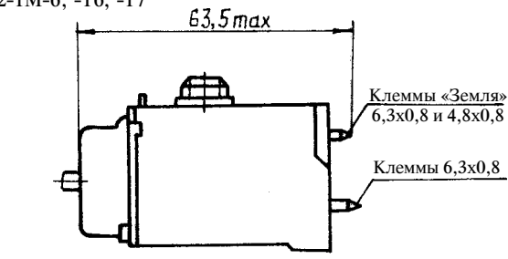
ТАМ112-1М-6, -16, -17
