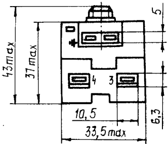
ТАМ112-1М-1, -3, -4, -60
