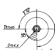
ТАМ112-1М-87
